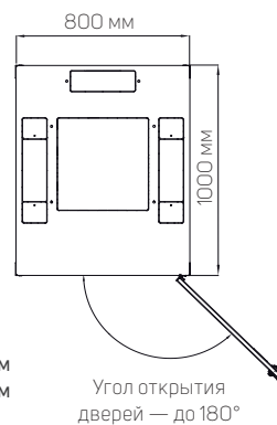
ПРИМЕР — УГОЛ ОТКРЫТИЯ ДВЕРИ
